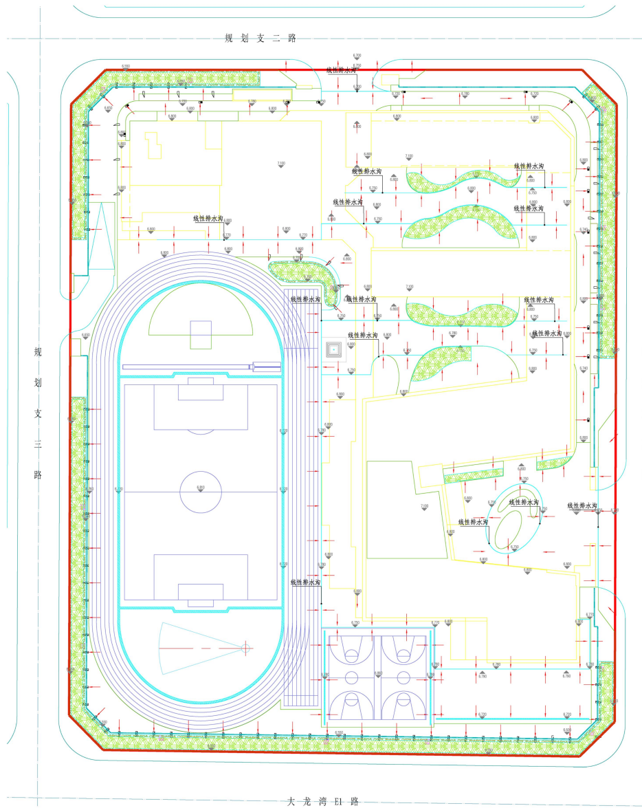
图 1.1-6 项目竖向布置图
